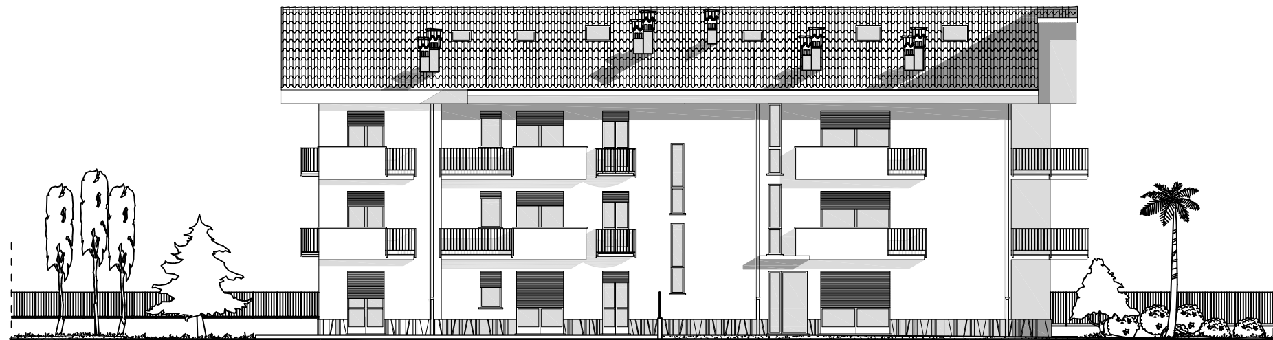
PROSPETTO OVEST
