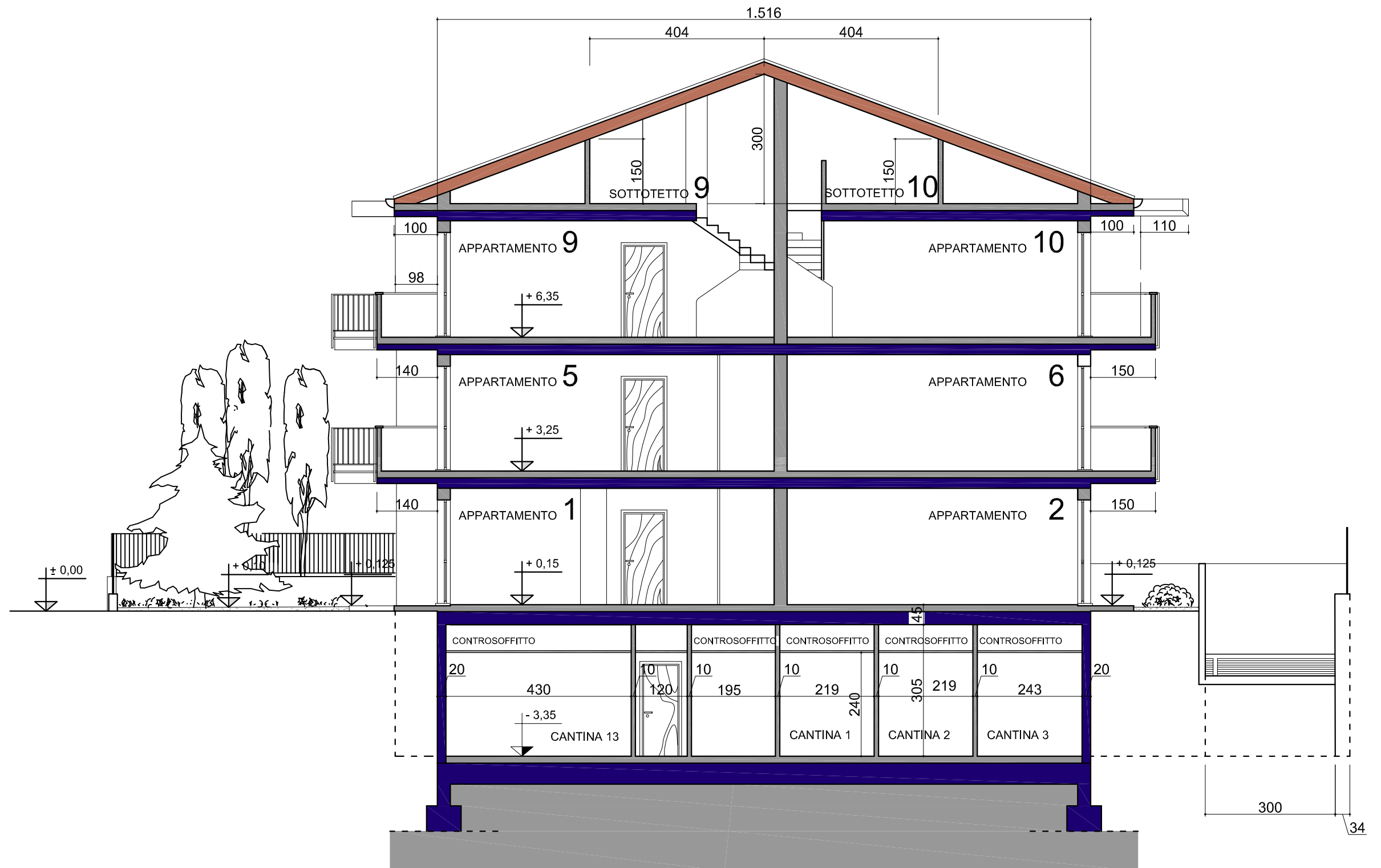
SEZIONE A - A' rapp. 1 : 50
