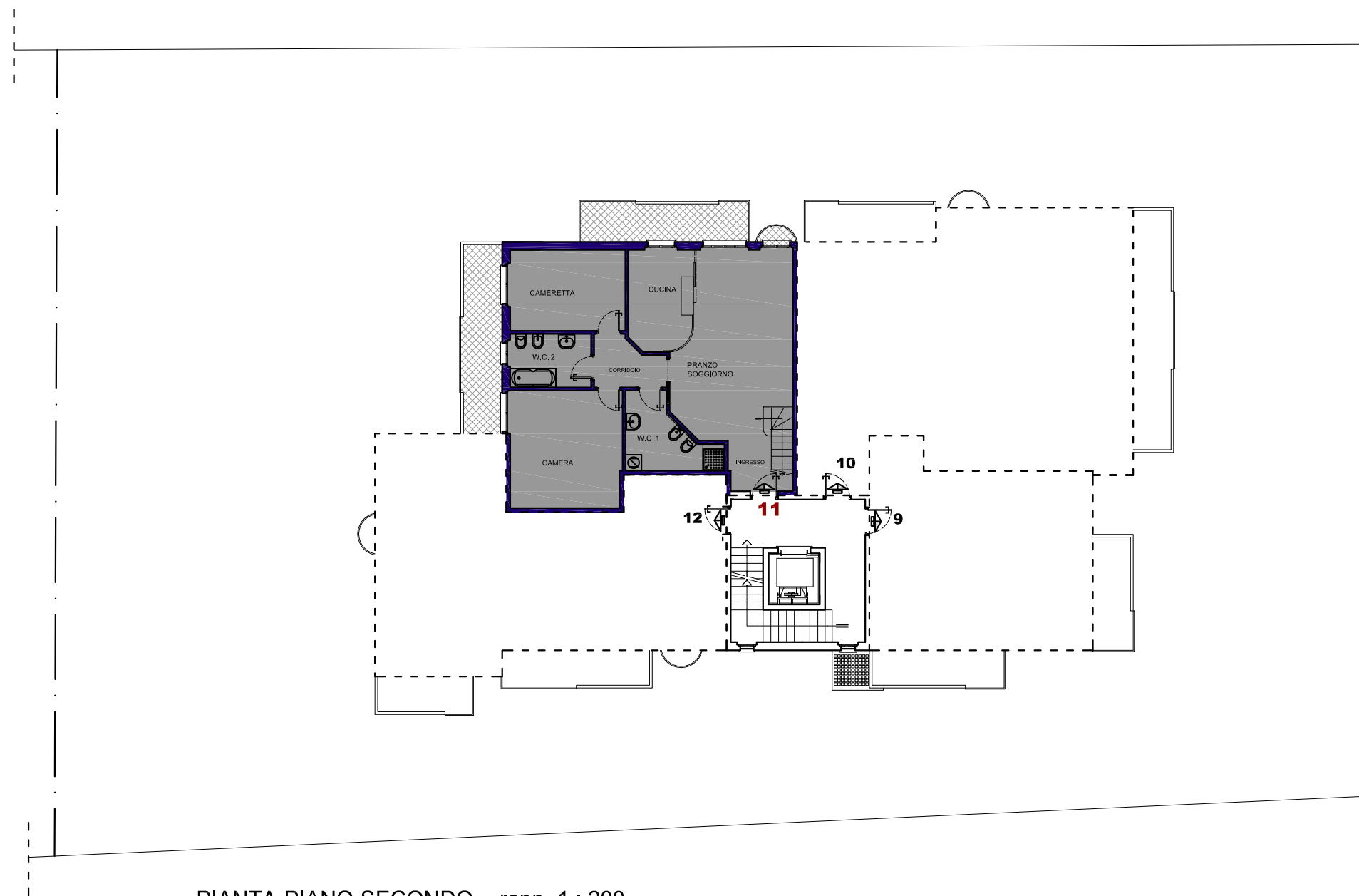
PIANTA PIANO SECONDO rapp. 1 : 200
