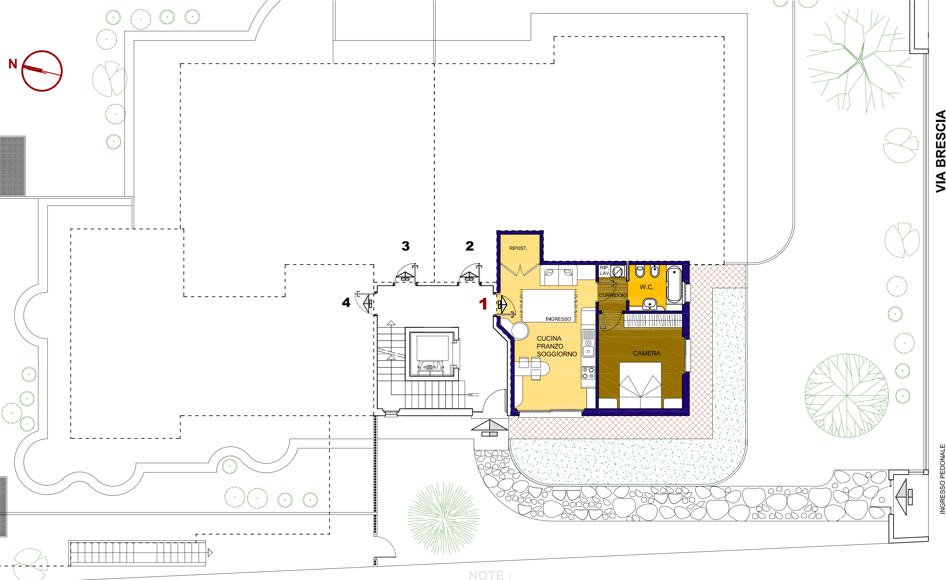
PIANTA PIANO TERRA rapp. 1 : 100
